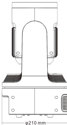
侧面图
