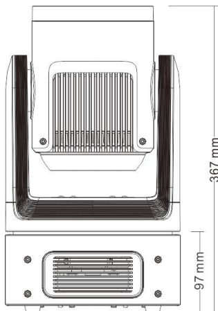
正面图
