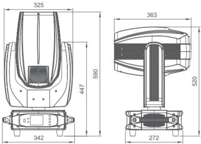
主视图
