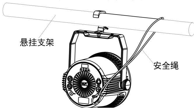
图（4.2-2）：安全绳安装图
