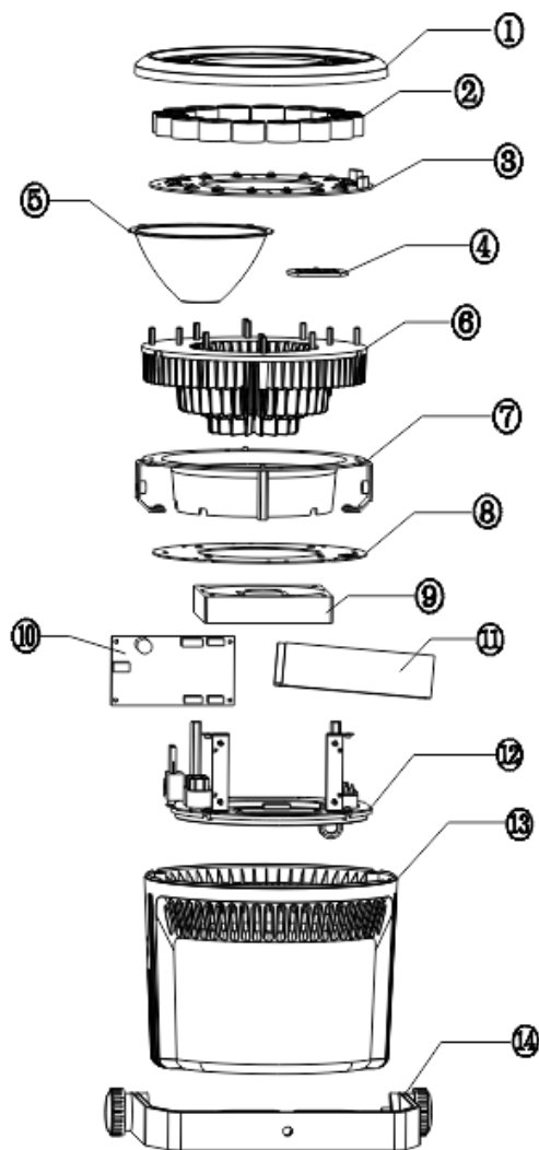
附 1：灯具结构分解图
