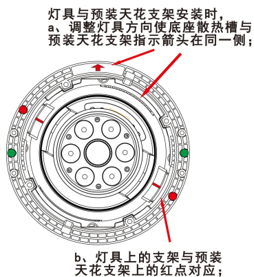
灯具与预装天花支架安装前对位情况
