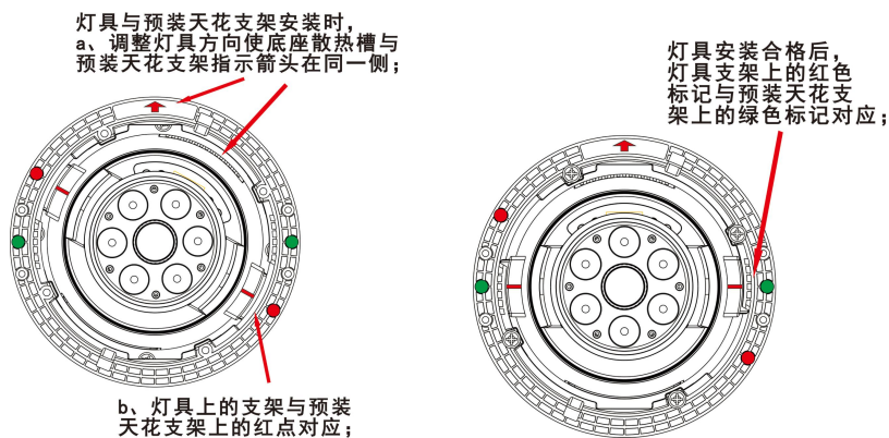
灯具与预装天花支架安装前对位情况
